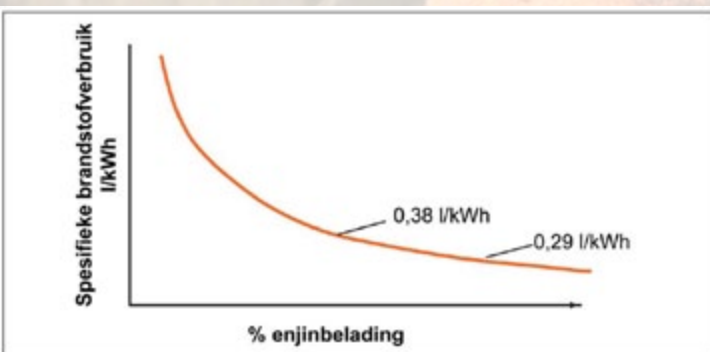
Grafiek 1: Verhoging in spesifieke brandstofverbruik met verhoging van enjinbelading.
