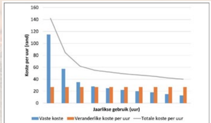
Grafiek 2: Eenheidstrekkerkoste met verhoging van jaarlikse gebruiksure.
